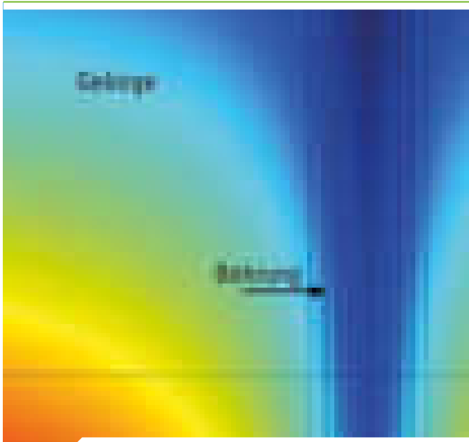
Kombiniertes Gebirgs- und Bohrungsmodell
